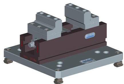
Mechanischer Zentrischspanner MZU auf Adapterplatte Mechanical centre-clamping vise MZU on adapter plate
