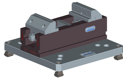
Mechanischer Zentrischspanner MZE auf Adapterplatte Mechanical centre-clamping vise MZE on adapter plate
