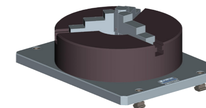
Dreibackenfutter DBF auf Adapterplatte Three jaw chuck DBF on adapter plate
